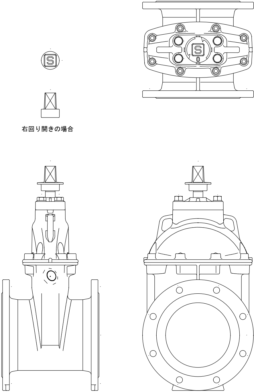
JWWA B 120 水道用ソフトシール仕切弁
