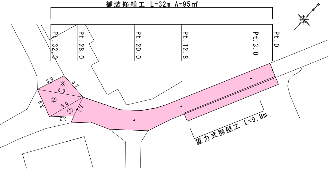
平面図 S=1:300
