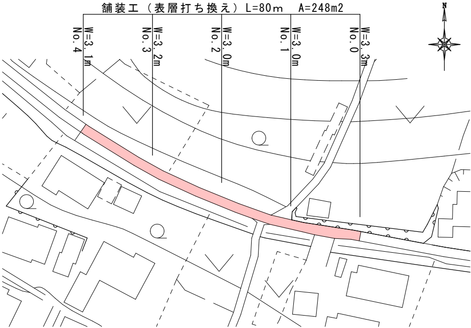
平面図 S=1:1000 (A4)
