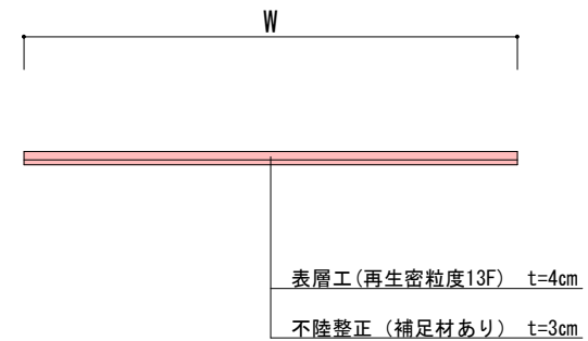
標準断面図 S=1:50 (A4)
