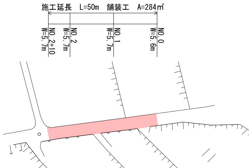
平面図 S=1:1000 (A4)
