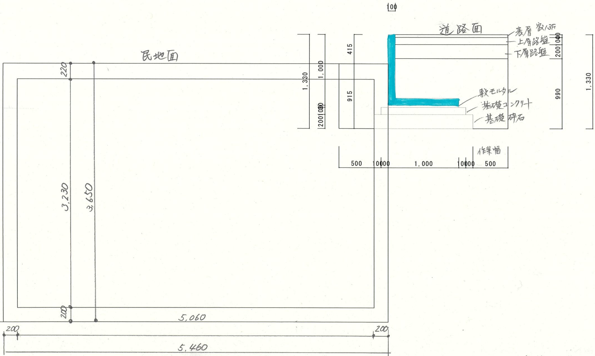
L型擁壁設置図
