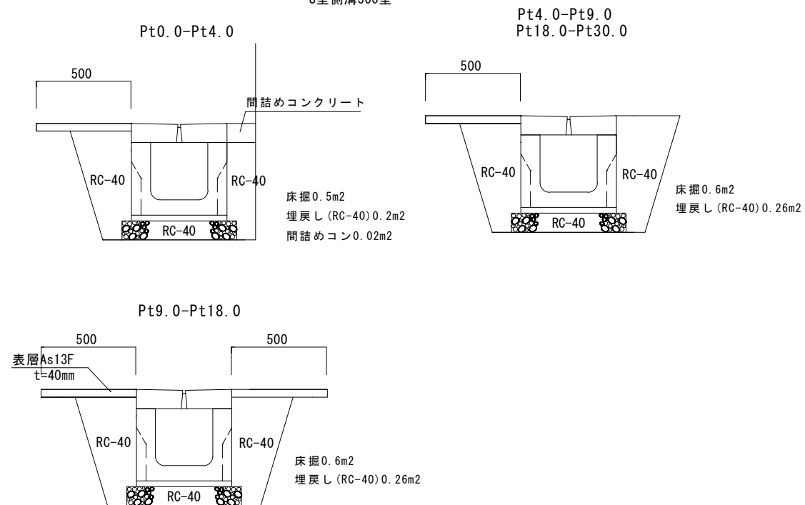
側溝断面 (縦断) S=1 : 20 U型側溝300型
