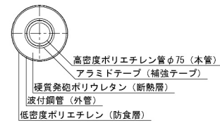
送水管構造図
