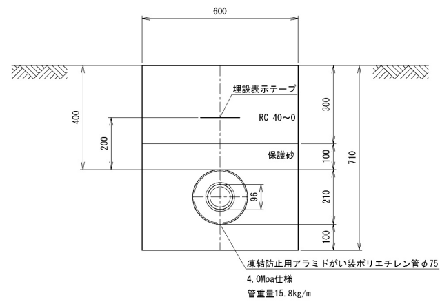
送水管構造図
