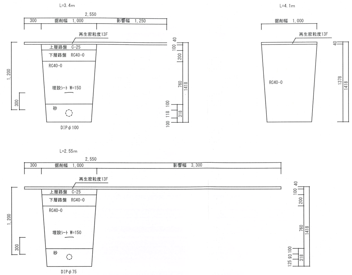
【 断面図 】 S=1/40
