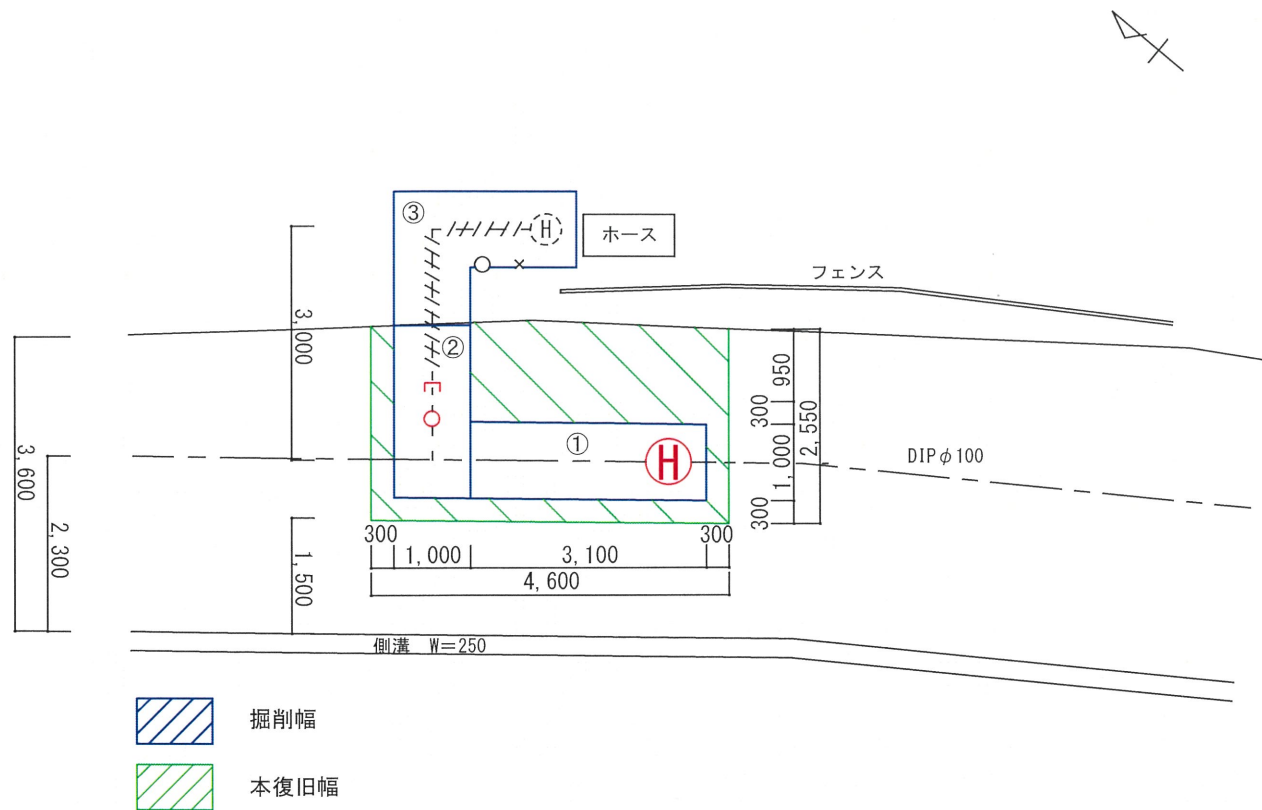
【 平面図 】 S=1/100
