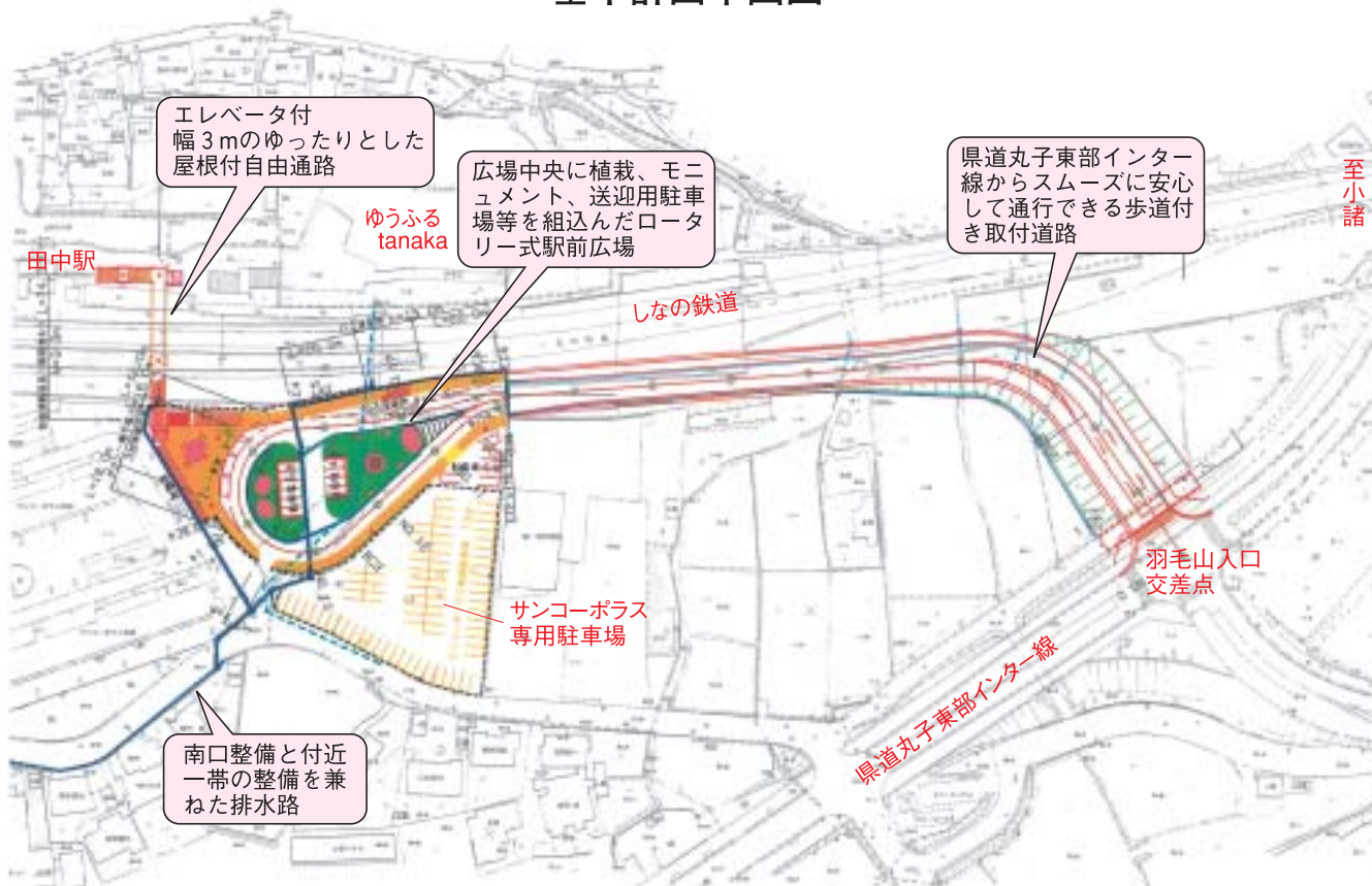
基本計画平面図
