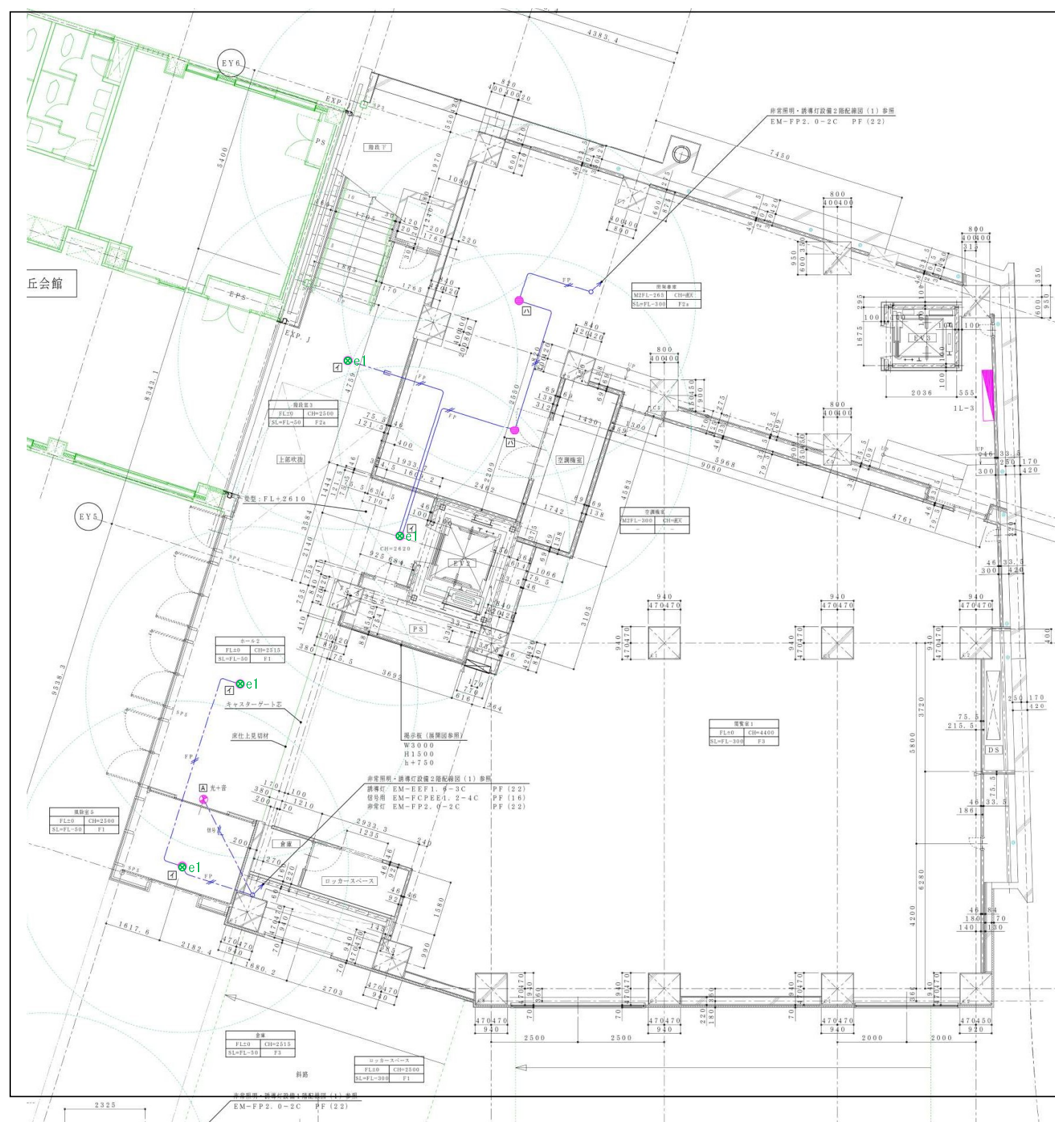
図書館 1階(通路・階段等) 改修平面図 * 非常灯改修
