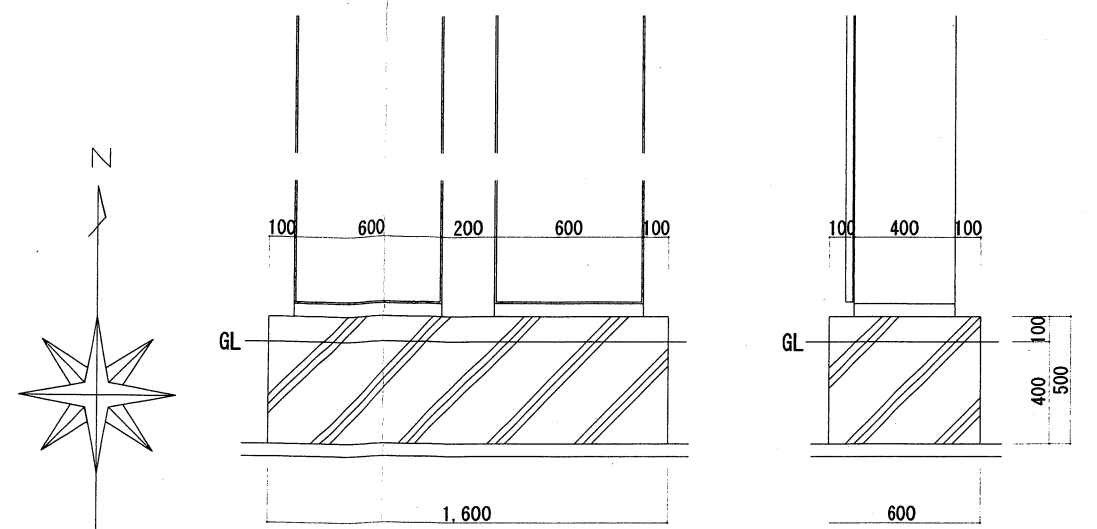
ポンプ制御盤・計装盤基礎図
