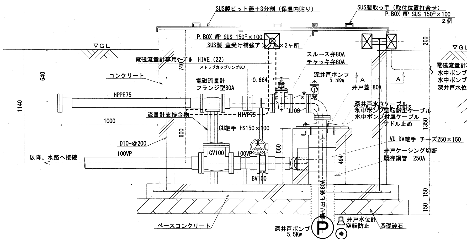
井戸ピット断面図 S=1/20
