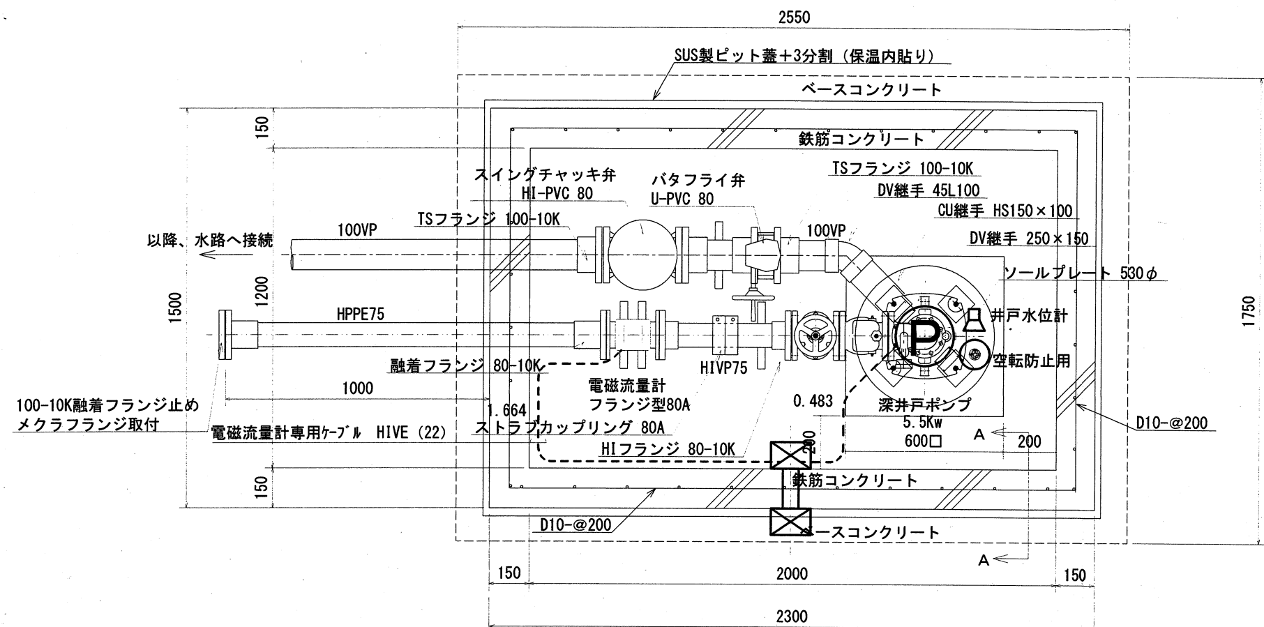
井戸ピット平面図 S=1/20
