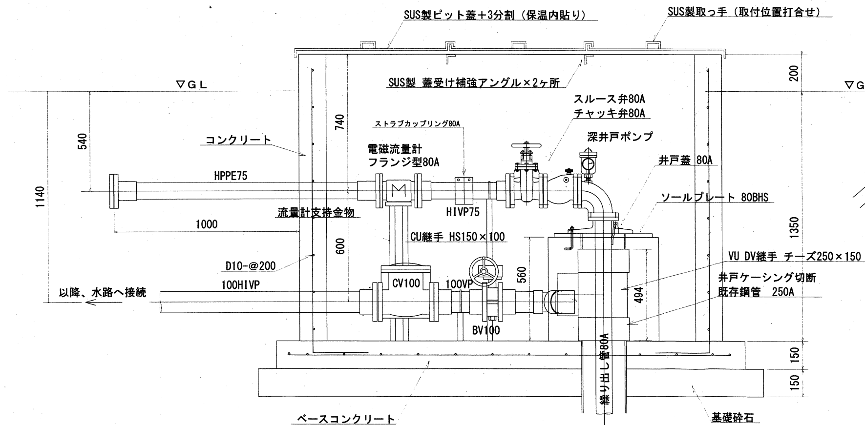
井戸ピット断面図 S=1/20
