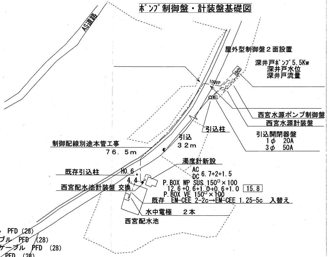
配置図 S=1/1000
