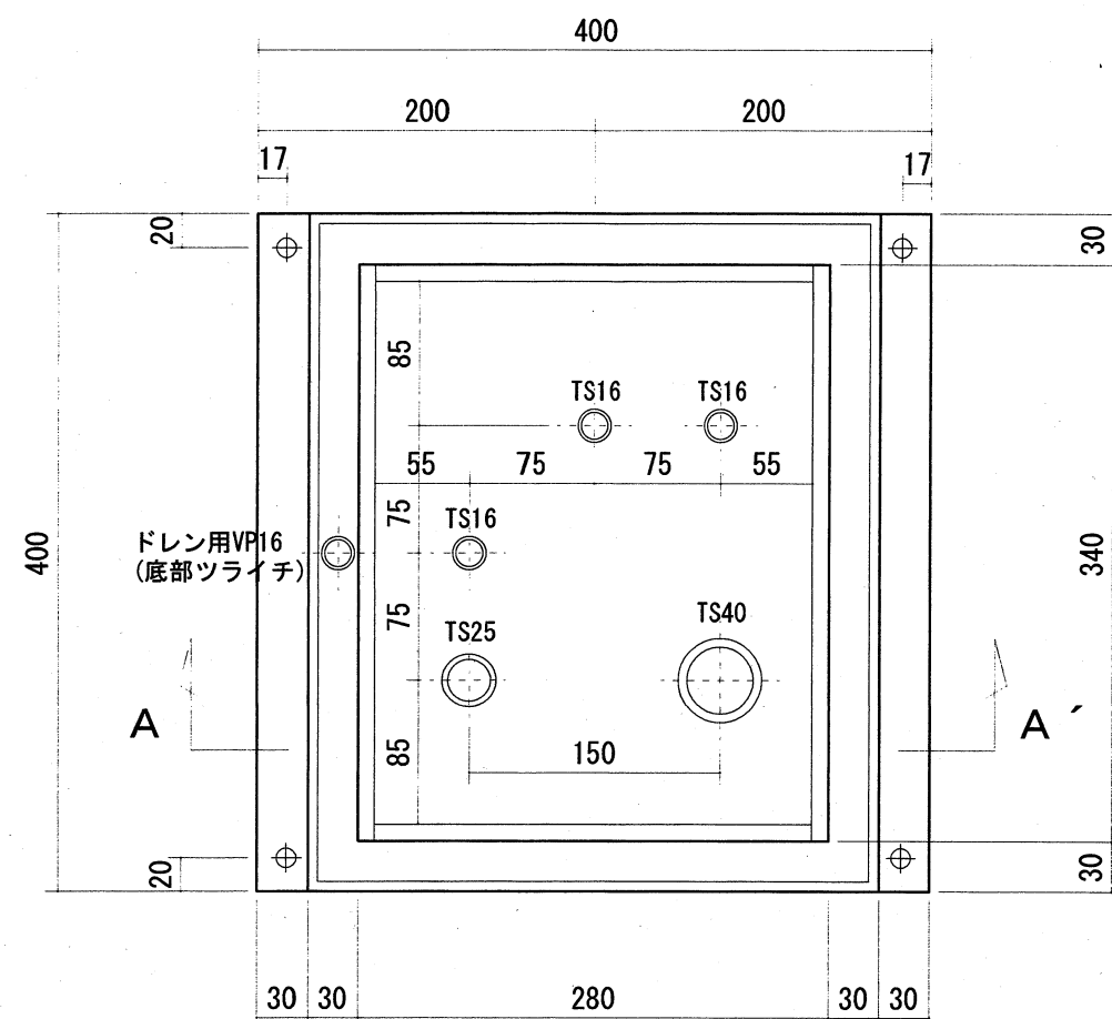
脱泡槽平面図 S=1/5
