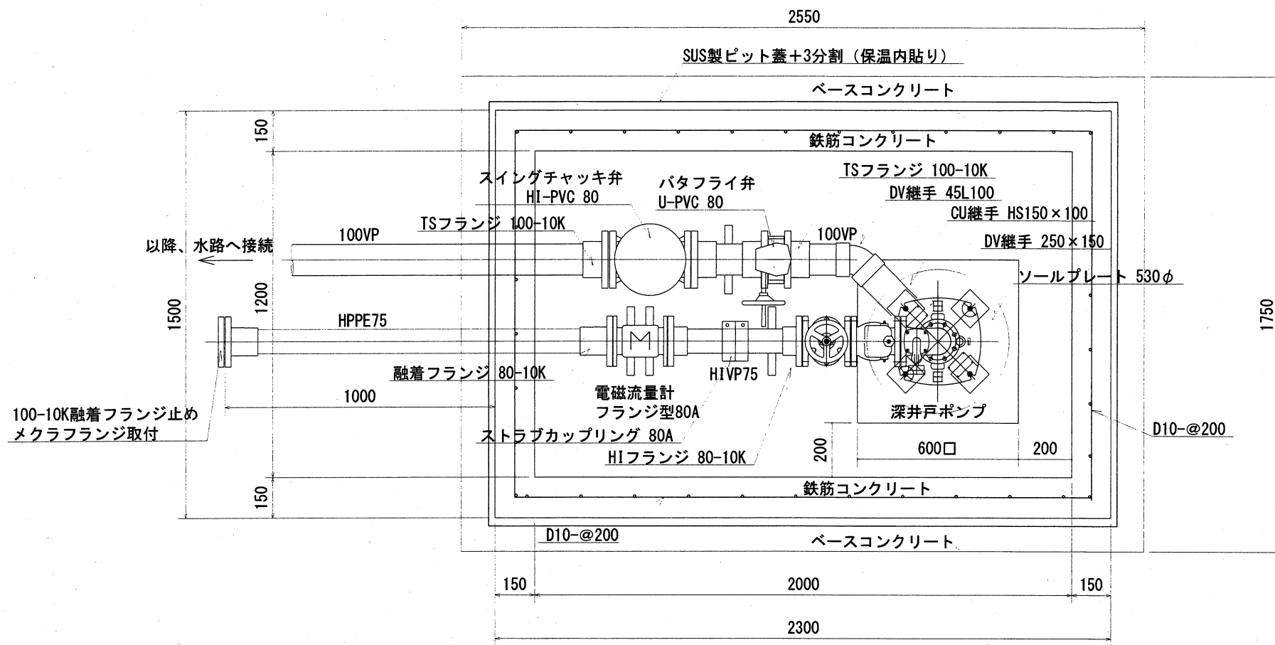
井戸ピット平面図 S=1/20
