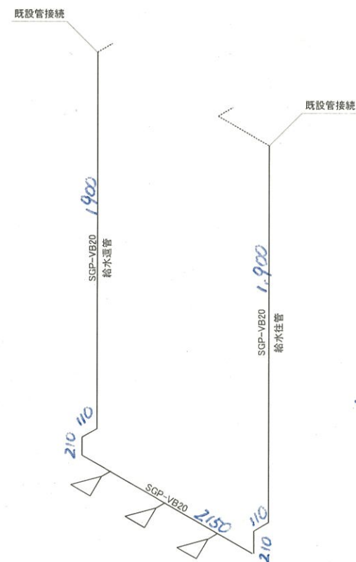
立面図
