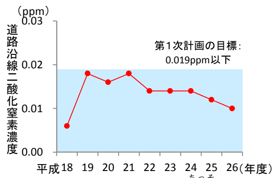
図 3-3 道路沿線二酸化窒素濃度の推移
