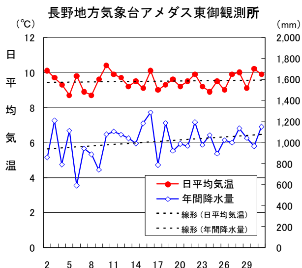
図 11 平均気温と降水量の推移
