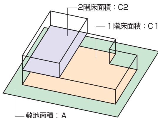
図2 容積率
